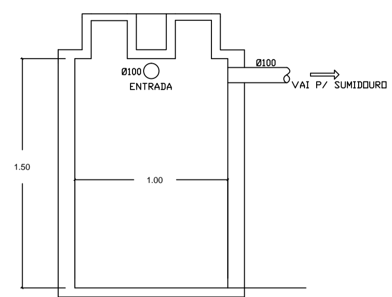
FOSSA Esc. 1:25
