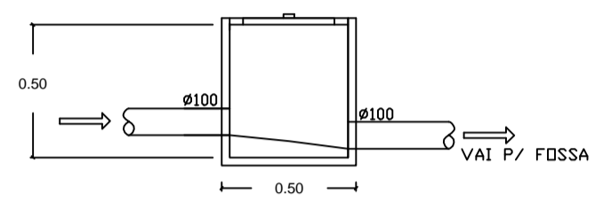
CAIXA DE PASSAGEM Esc. 1:25
