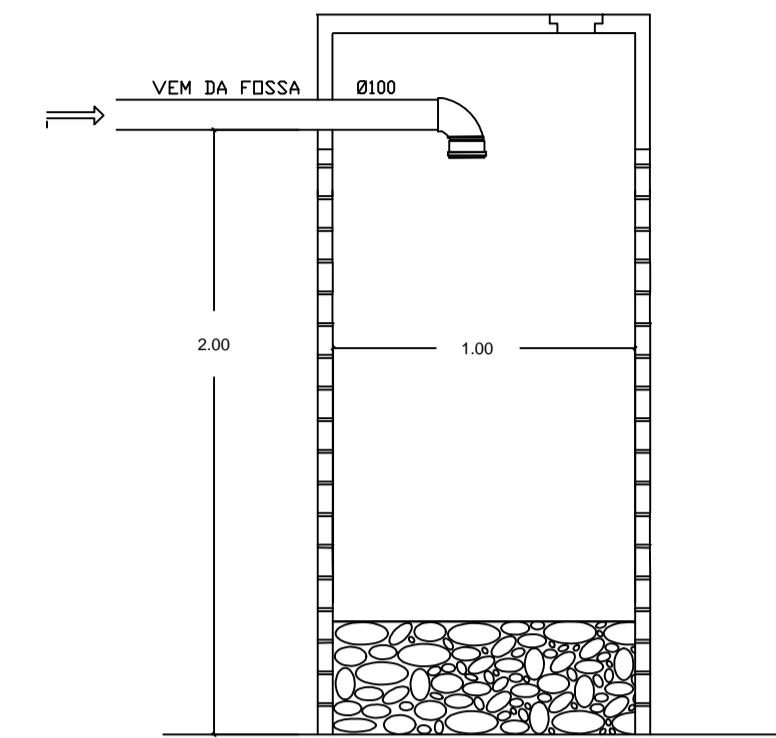
SUMIDOURO Esc. 1:25
