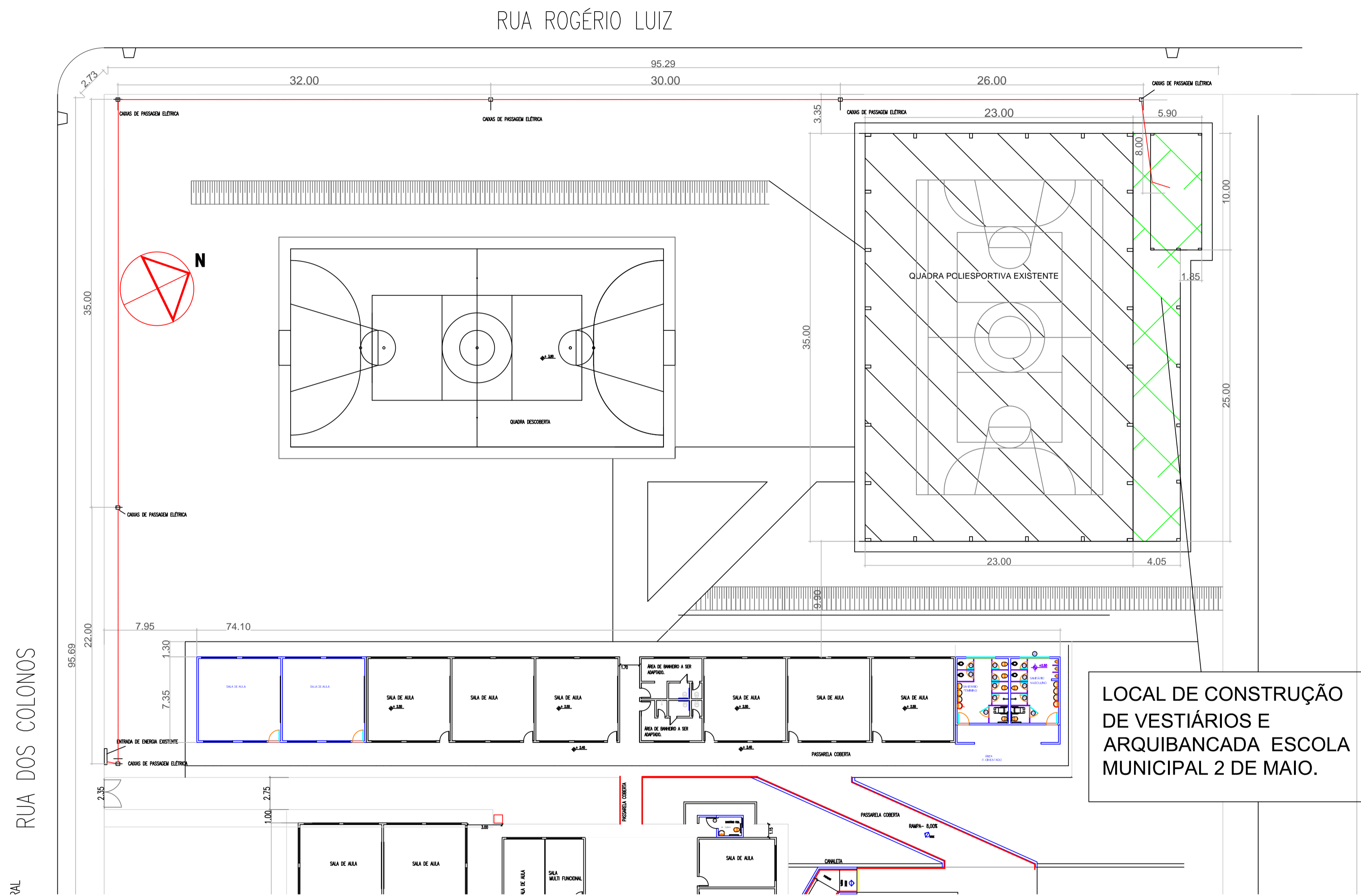
INSTALAÇÕES ELÉTRICAS LOCAÇÃO DAS CAIXAS DE ENERGIA E PADRÃO DE ENTRADA. Esc. 1:250
