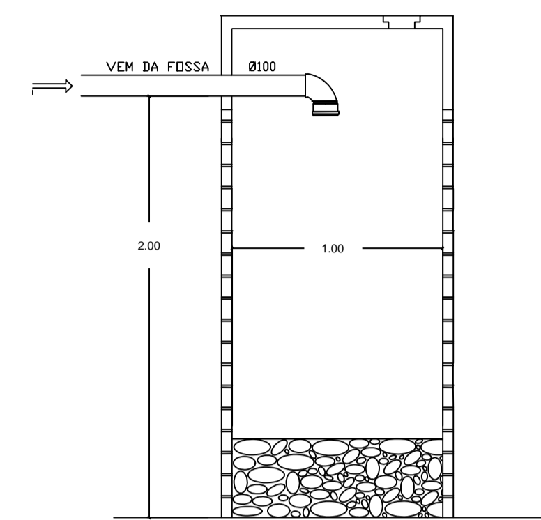
SUMIDOURO Esc. 1:25
