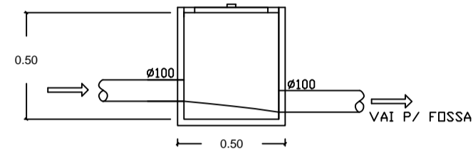
CAIXA DE PASSAGEM Esc. 1:25
