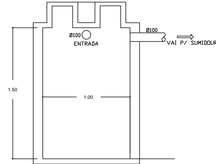
FOSSA Esc. 1:25
