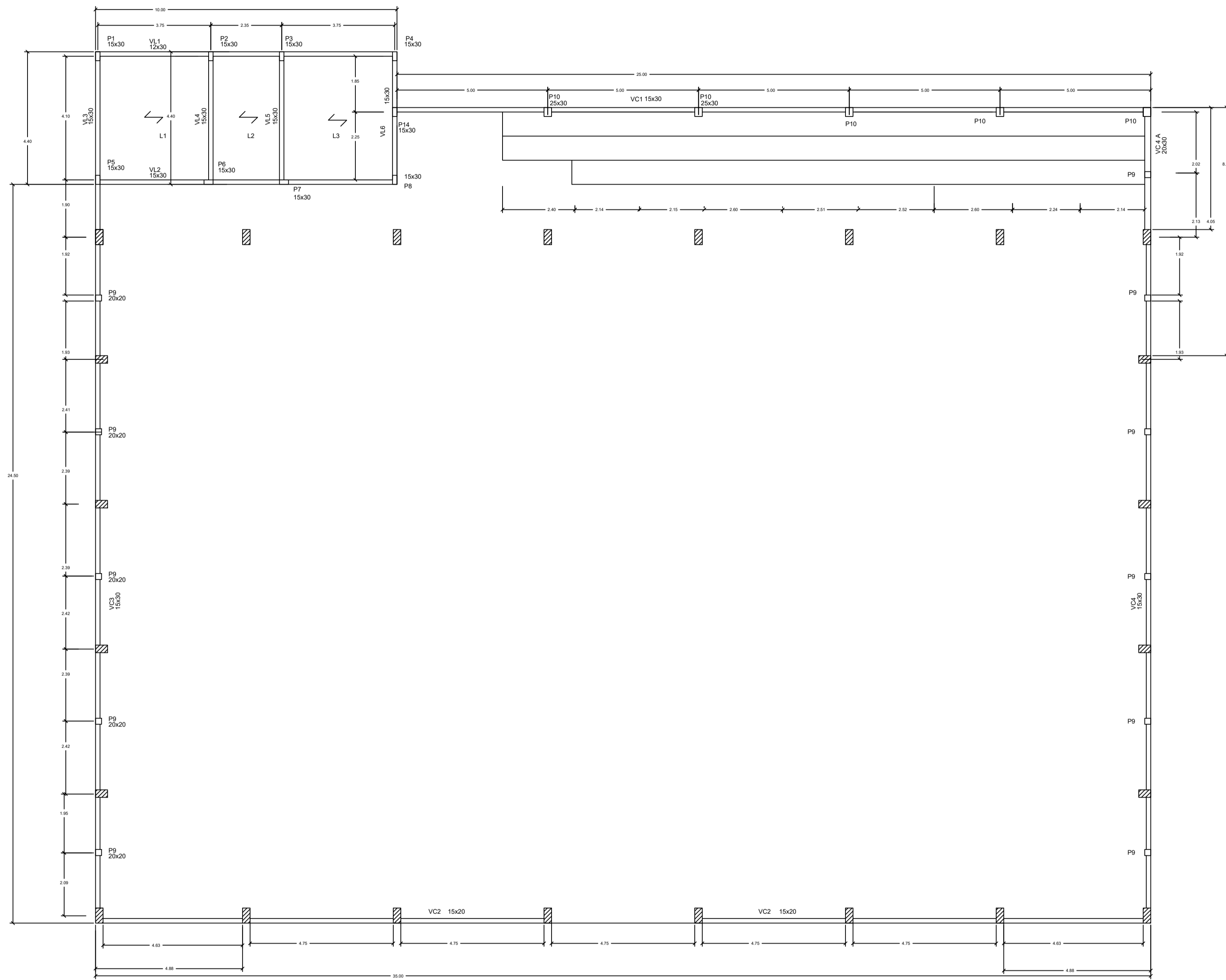
FORMA VIGAS DA LAJE E FECHAMENTO Esc. 1:100
